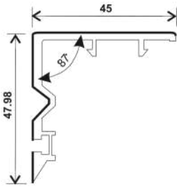
T-MFB(I), INTERLOCK DOOR (45*48)
