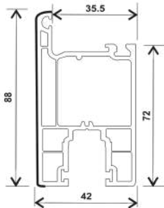
R T-MS, SLIDING DOOR SASH (42*88) 1.193
