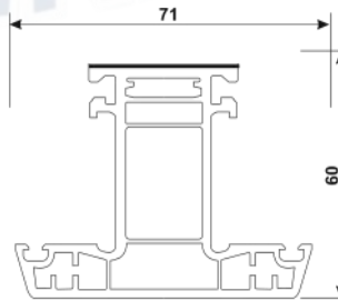
R P60-ZT-D, MULLION T CASEMENT (60*71) 1.198
