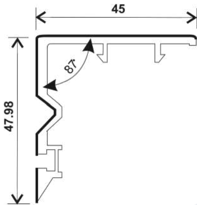
R T-MFB(1), INTERLOCK DOOR (45*48)
