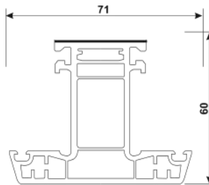
P60-ZT-D, MULLION T CASEMENT (60*71)
