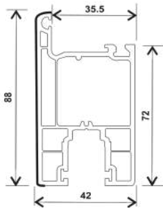
T-MS, SLIDING DOOR SASH (42*88)
