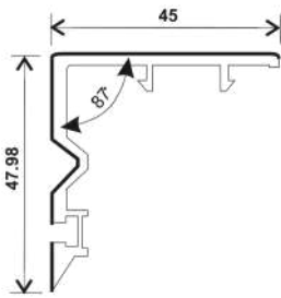
T-MFB(I), INTERLOCK DOOR (45*48)
